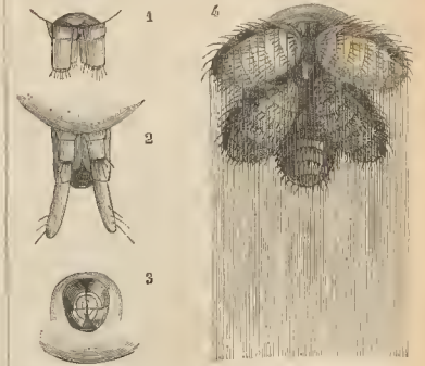
Fig. 3. Hileras. - 1. En haz. - 2. Palpiforme. - 3. En roseta cerrada. - 4. La misma abierta y muy aumentada: en ésta se ven los hilos paralelos antes de unirse.
